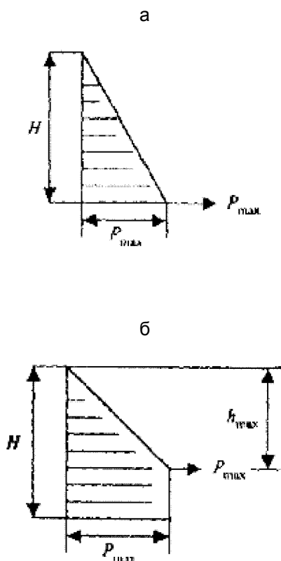
Рисунок 16.1. Расчетные эпюры бокового давления бетонной смеси
